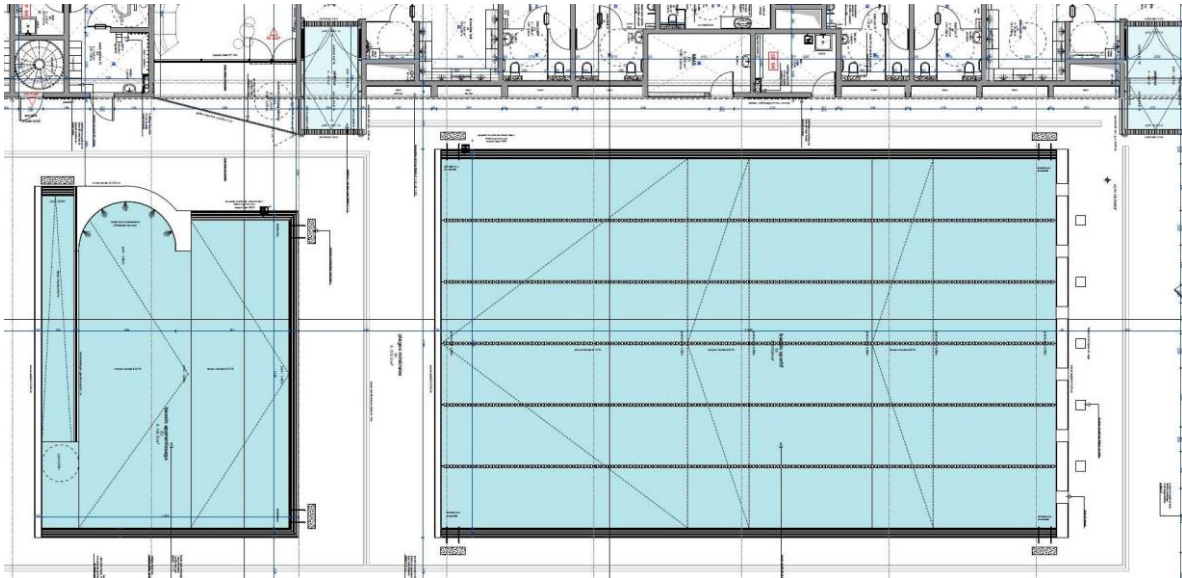
Plan de coupe des bassins :
